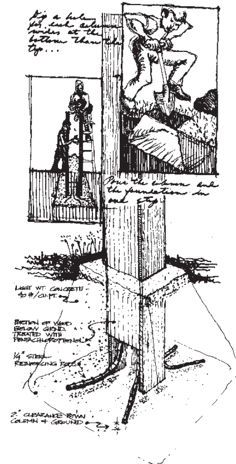
Eine Version von Wurzelfundierung für einen hohlen hölzernen Kastenpfeiler, den wir gebaut haben.
